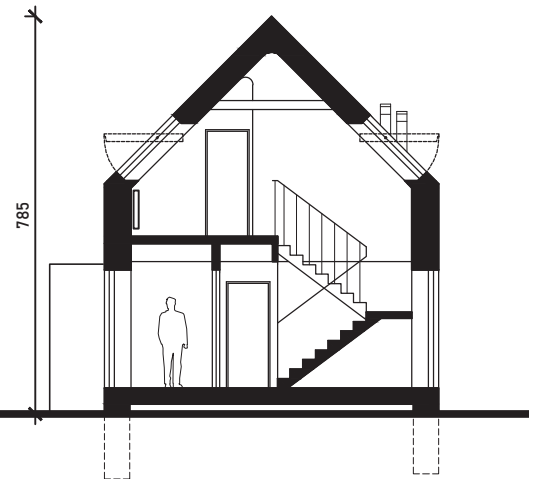
PRZEKRÓJ
