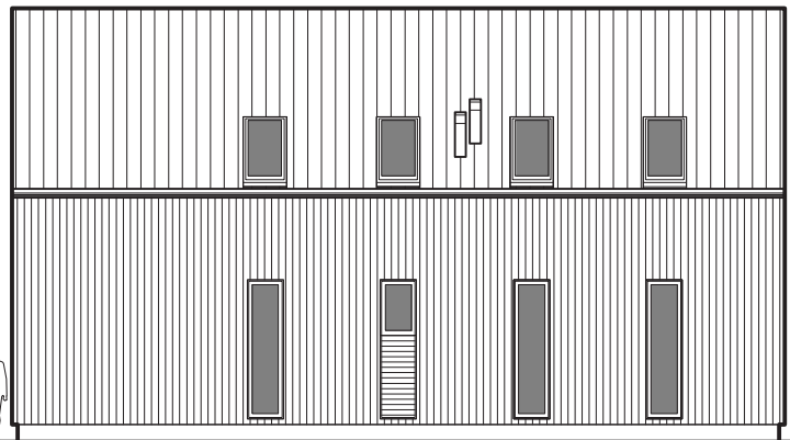
ELEWACJA WSCHODNIA
