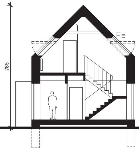
PRZEKRÓJ
